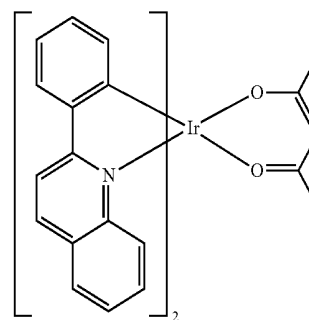
Ir(pq) 2 (acac)
